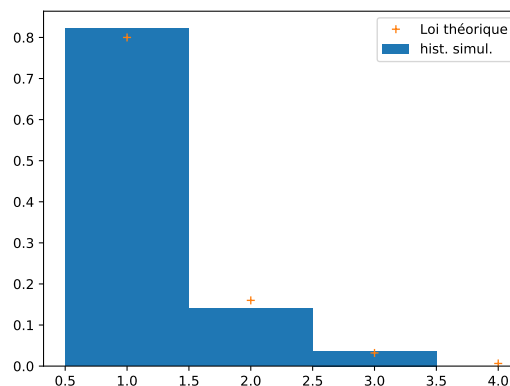
(b) Une simulation et la loi théorique NS = 300 tirages, p = 0.8
