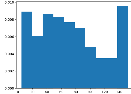
(b) Distribution temps de sortie : Le jeu est fini en moins de 151 tours dans 90% des cas.
