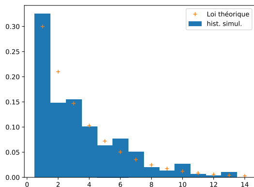
(a) Une simulation et la loi théorique NS = 300 tirages, p = 0.3
