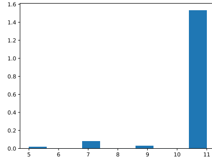
(b) Distribution temps de sortie : Au bout de 10 tours, le jeu n'est dans la plupart des cas pas fini
