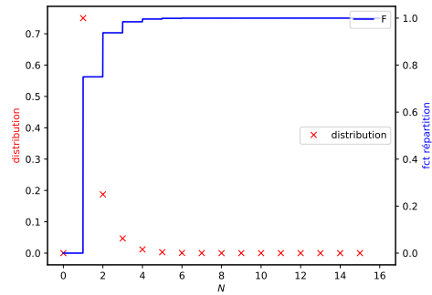
(d) Distribution géométrique, p = 0.75
